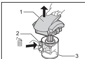
1. Couvercle 2. (P) bouton 3. Contenant à poussières
